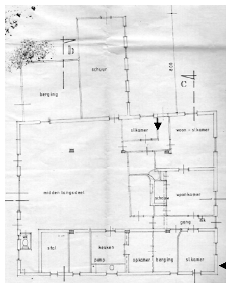
Plattegrond uit 1991. De schuur en berging aan de oost kant zijn ooit aangebouwd. De pijltjes staan bij de voordeuren van A159 en A160.
